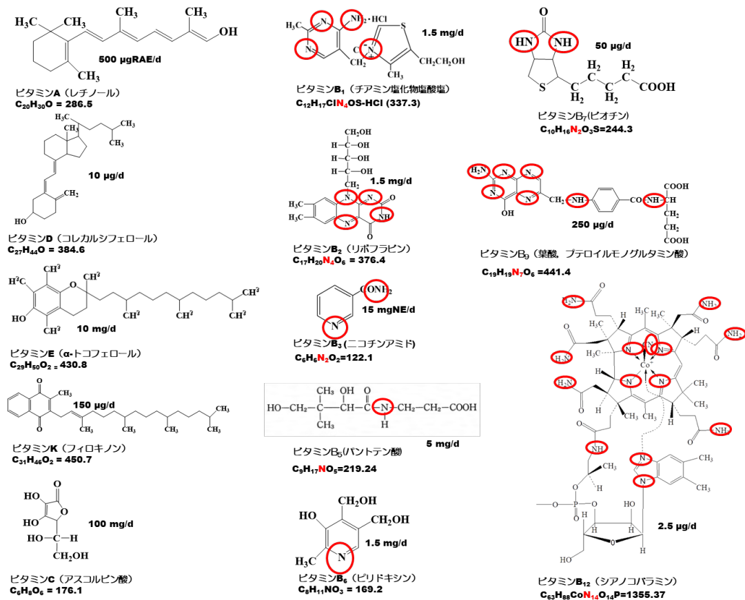
図3. ビタミンの構造式
